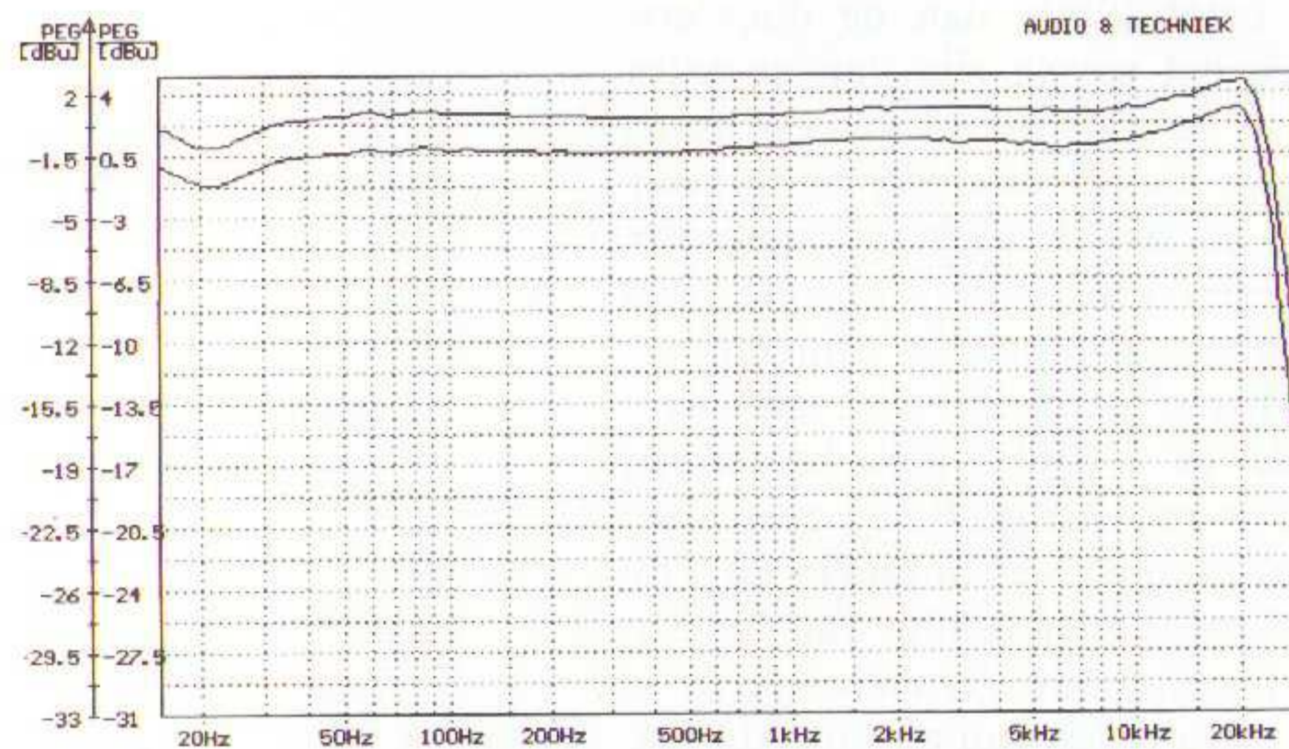
Sony TC-K770ES
